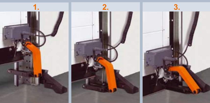
Боковой отбойник препятствует повреждению кронштейнов опережающего светового барьера в закрытом положении ворот.
